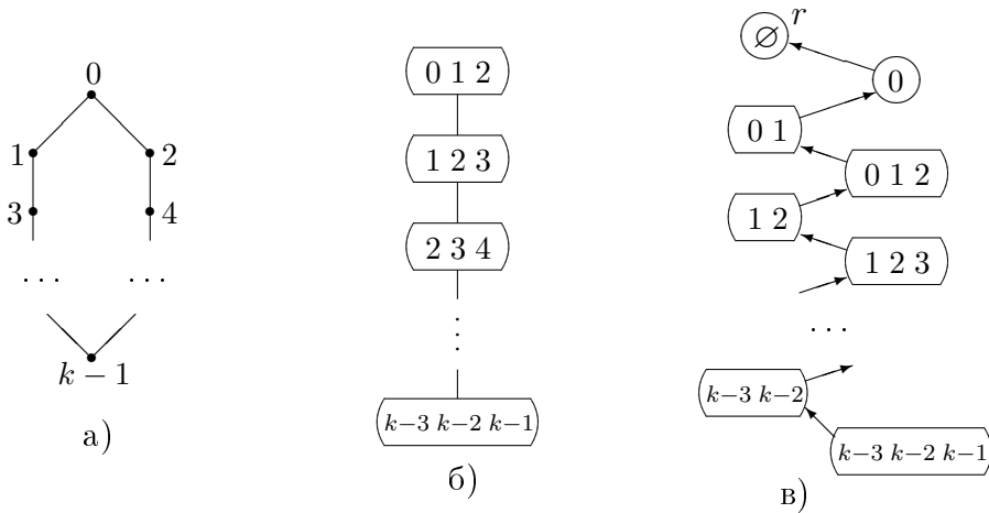
Рис. 11.1: Граф \mathcal{C}_k (а), его древесное разложение (б) и приведенное древесное разложение (в).
