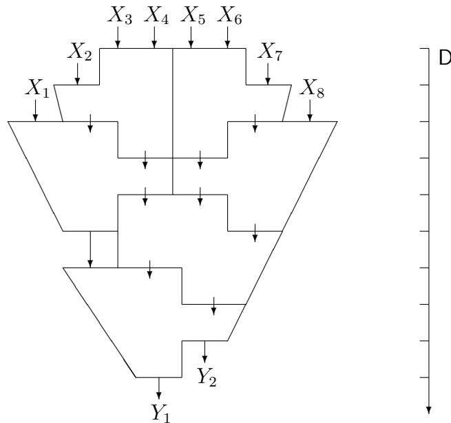
Рис. 4.1: Схема многократного сложения из (3, 2) -компрессоров [279]
