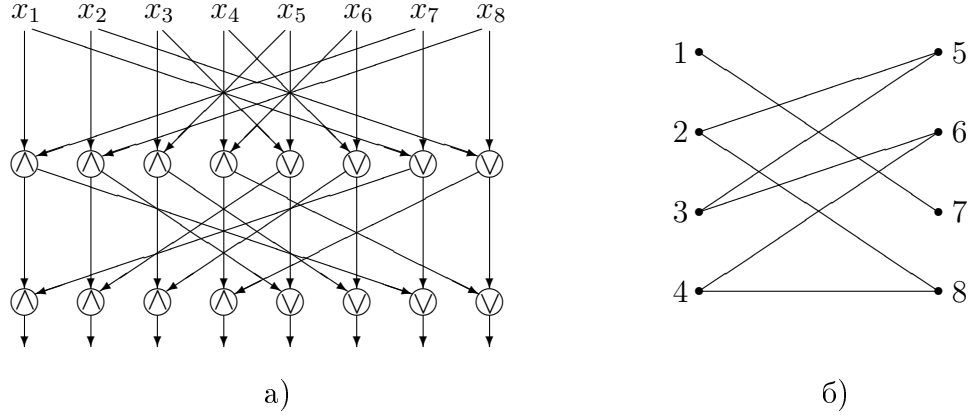
Рис. 5.1: Схема компараторов и ее граф
