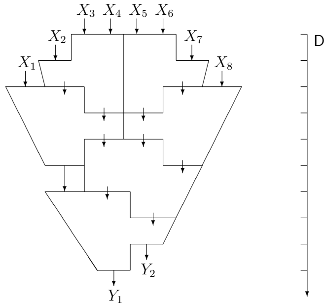
Рис. 4.1: Схема многократного сложения из (3, 2)-компрессоров [299]
